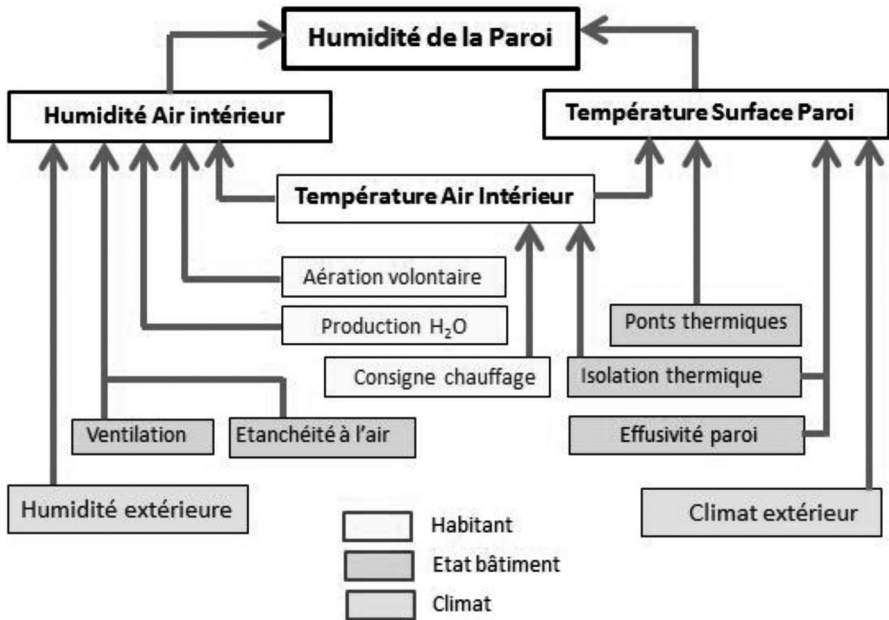
FIG. 1. — Principaux éléments conditionnant le taux d'humidité intérieure d'un logement [22]
