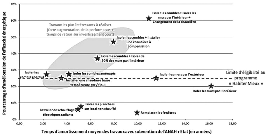
FIG. 2. — Classement des interventions sur le bâtiment en fonction du pourcentage d'amélioration de l'efficacité énergétique et du temps d'amortissement moyen des travaux
